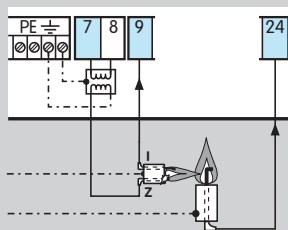
BCU 480..P с промышленным штекером Обозначения на схеме - смотри Обозначения.
