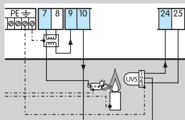
BCU 480..P с промышленным штекером Обозначения на схеме - смотри Обозначения.
